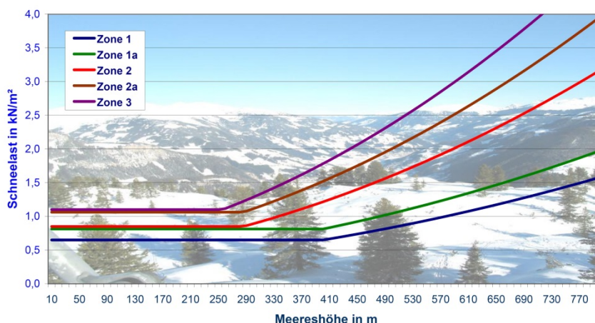
Abbildung 2: Schneelastzonenkarte, Quelle: www.wikipedia.de
