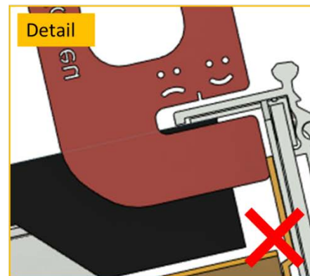
Einkerbung Haltekante
