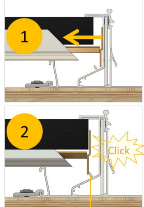
Rastkante
